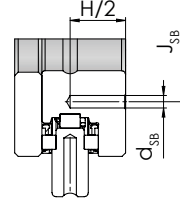
C-C (1x sensor bore)
